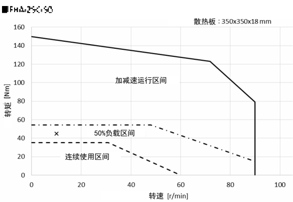
FHA-25C-50 可用区间
