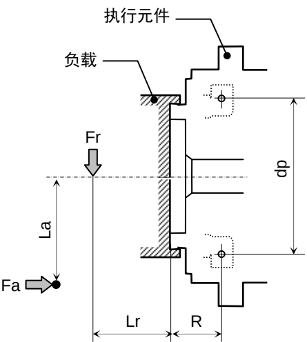
图 1: 外部负载作用图
